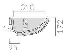
Sezione Section
