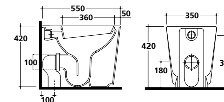
5409NE Vaso con scarico universale "S/P, trasformabile tramite curva tecnica, nero. Fissaggio incluso. W.c. with floor/wall draining, adjustable by elbow/wall pipe, black. Fixing kit included. Inodoro para tanque alto salida horizontal ó vertical. Transformable por medio del sifón de evacuación, negro. Fijaciones incluidas.
