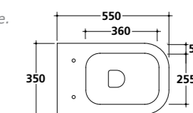
5409 Vaso con scarico universale "S/P, trasformabile tramite curva tecnica. Fissaggio incluso. W.c. with floor/wall draining, adjustable by elbow/wall pipe. Fixing kit included. Inodoro para tanque alto salida horizontal ó vertical. Transformable por medio del sifón de evacuación. Fijaciones incluidas.
